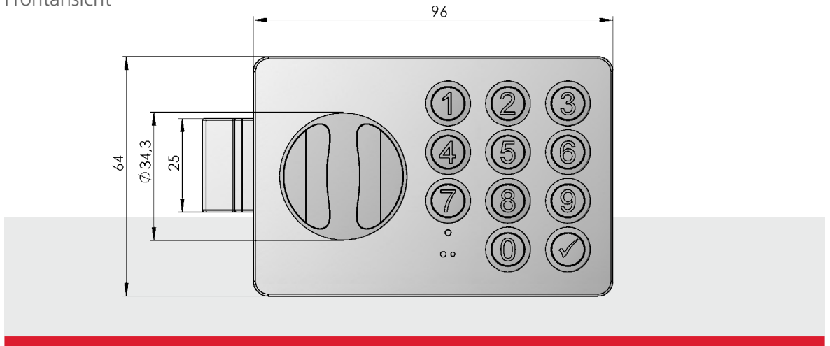
Frontansicht
